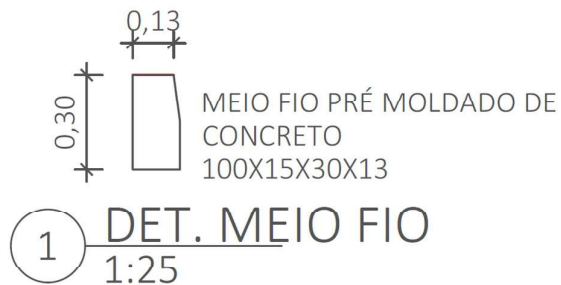
Figura 1: RECORTE DA PLANTA (SEM ESCALA)
