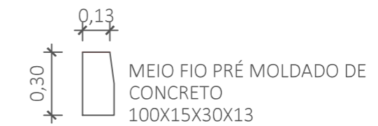
1 DET. MEIO FIO 1:25
